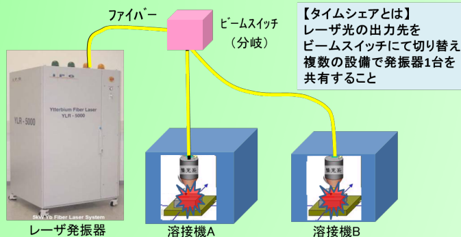
タイムシェアによる溶接サイクル(イメージ)
