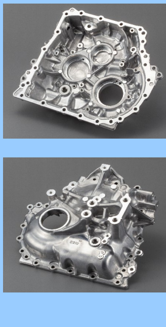
eAxleユニット部品
